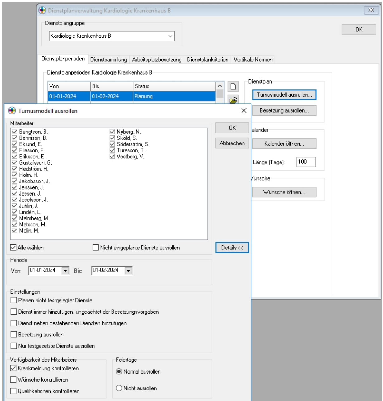
Abbildung 2.6: Neue Dienstplanperioden können das Turnusmodell nutzen, indem es ausgerollt wird.
